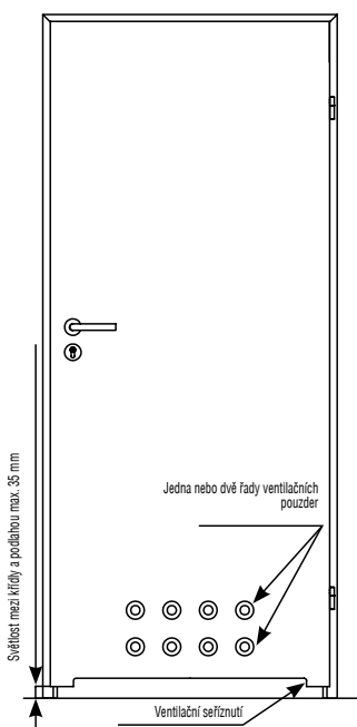
ventilační seřiznutí v bezalcových křídlech z kolekce FIESTA '09 střihané DUO - příplatek 589
