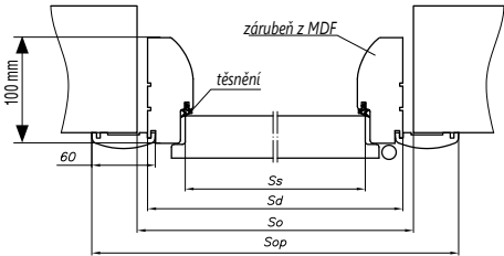
dveře s pevnou zárubní
