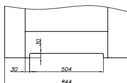
ventilační seřiznutí v křídlech ARCO „80“
