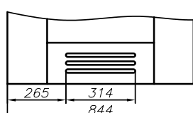
křídlo SEMPRE „80“ s ventilační mezerou
