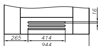
křídlo SEMPRE „90“ s ventilační mezerou
