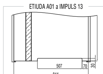
ventilační seřiznutí v křídlech Etiuda A01 „80“ a Impuls 13 „80“ - příplatek 589
