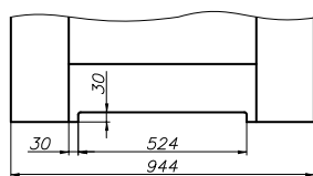
ventilační seřiznutí v křídlech SEMPRE „90“
