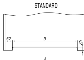
ventilační seřiznutí - příplatek 589
