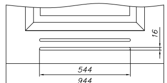
křídlo VERTIGO „90“ s ventilační mezerou
