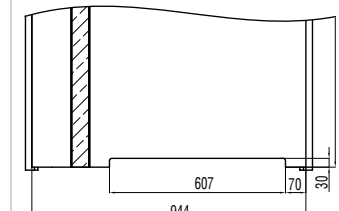
ventilační seřiznutí v křídlech Etiuda A01 „90“ a Impuls 13 „90“ - příplatek 589
