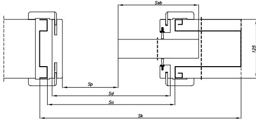
Varianta II – Tabulka II
