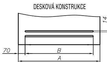
ventilační mezera v křídlech s deskovou konstrukcí – příplatek 589
