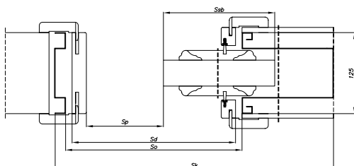
Varianta III – Tabulka III
