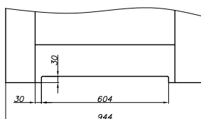
ventilační seřiznutí v křídlech ARCO „90“
