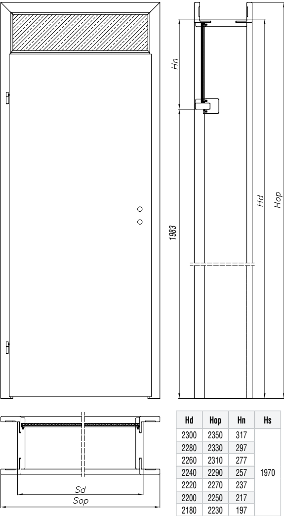
KOMPAKTNÍ SVĚTLÍKY SE ZÁRUBNÍ DIN
