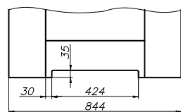
ventilační seřiznutí v křídlech SEMPRE „80“
